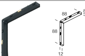
jonction en L plafond/mur pour Omnitrack MICRO P
