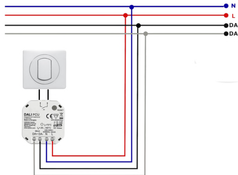
Module DALI
