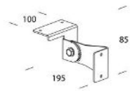
537 Étrier orientable
